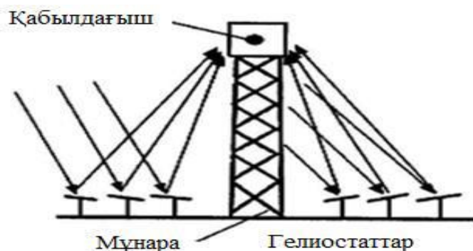
1 сурет - Мұнара типті күн электр станцияның ұстанымдық сұлбасы
