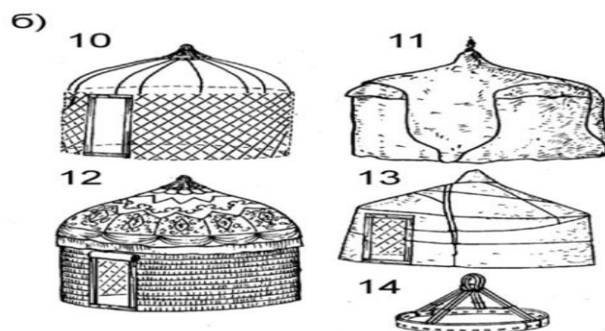
Рисунок 2. – Классификация мобильных сооружений (по С.И. Вайнштейну) б) юрты древнетюркского периода: 10 – реконструкция остова; 11 – внешний вид юрты монгольской знати в конце XIII – начале XIV вв. (реконструкция); 12 – юрта из Эджен-Хоро, т. н. «Усыпальница Чингисхана», Внутренняя Монголия; 13 – юрта хазарейцев, XX в.; 14 – перекрытие ее светодымового отверстия.
