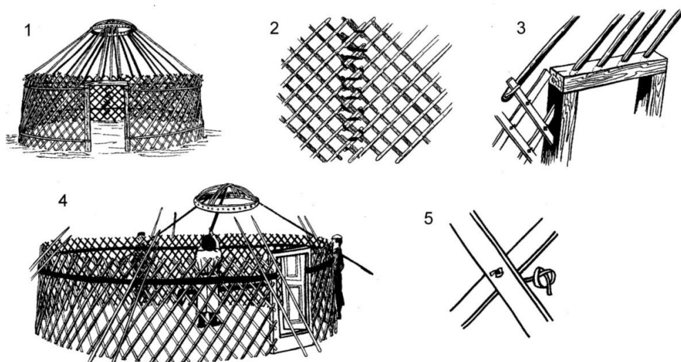
Рисунок 3. – Конструкция юрты и ее установка 1 – остов, 2 – соединение звеньев решетки, 3 – дверной косяк, 4 – скрепление планок решетки, 5 – установка остова.
